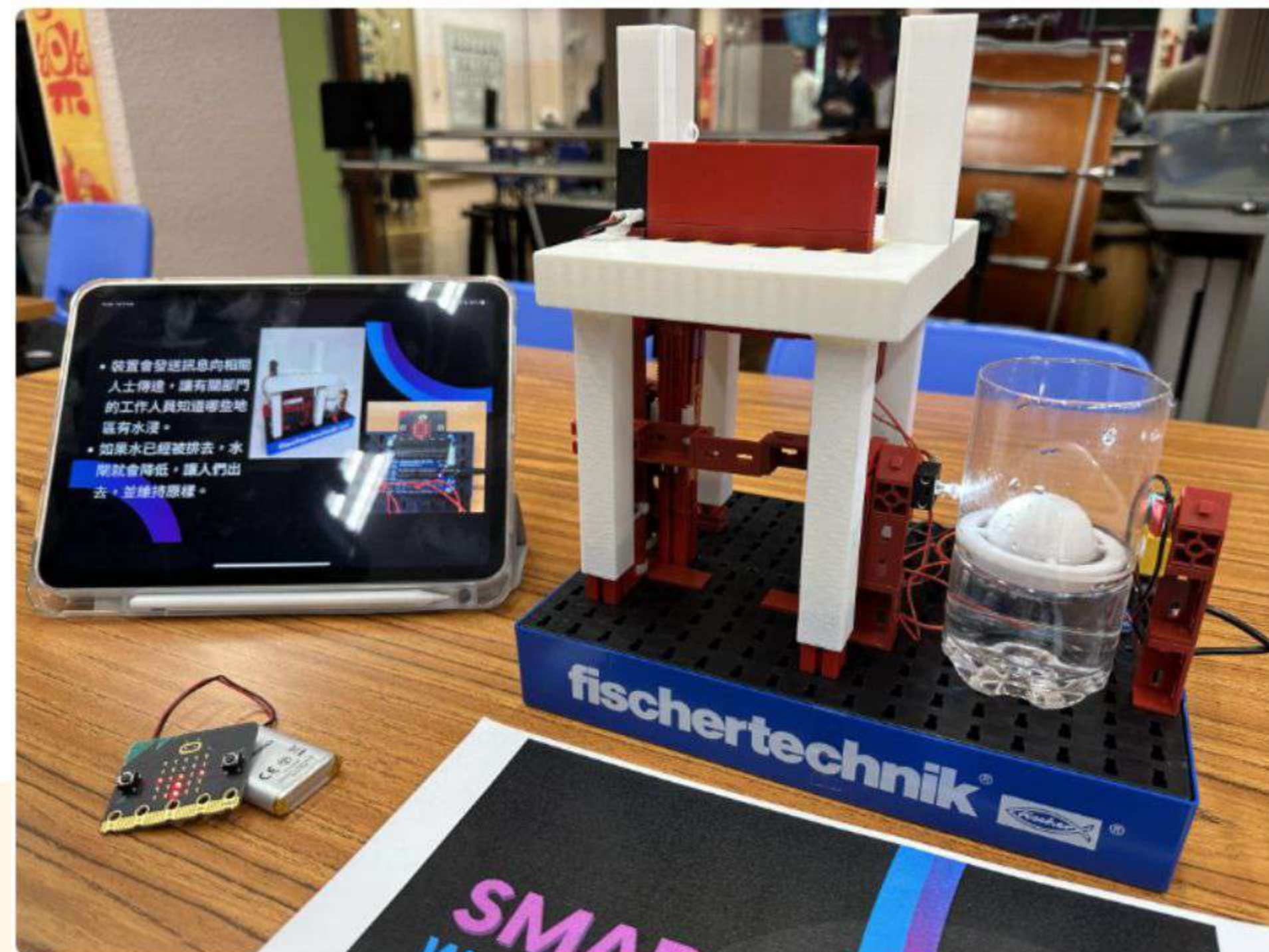
當暴雨令水位上升，感應球便會浮起，遮擋光線射向感應器，令水閘自動升起。
